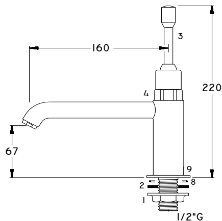
DIMENSIONES GENERALES
