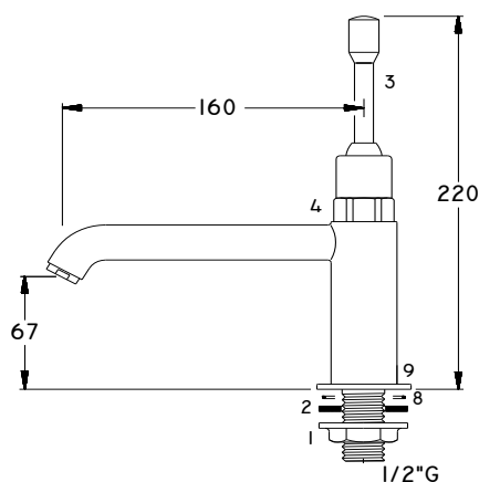
DIMENSIONES GENERALES
