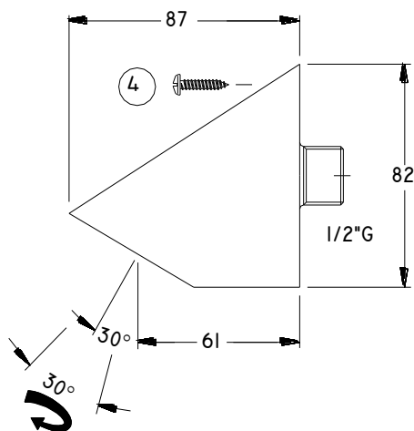
DIMENSIONES GENERALES Y COMPONENTES
