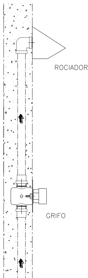
ESQUEMA TIPICO DE INSTALACION
