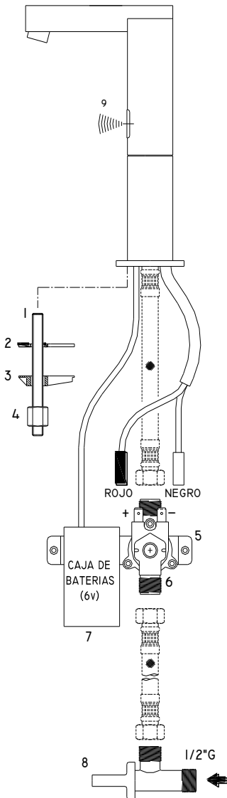
ESQUEMA DE CONEXIONES (ELECTRICA & HIDRAULICA)
