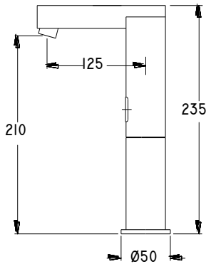
DIMENSIONES GENERALES
