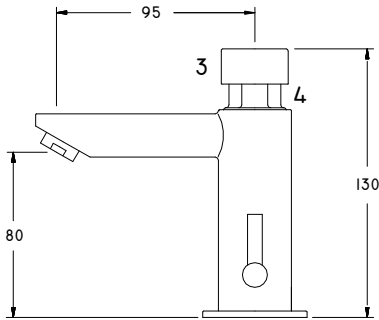
DIMENSIONES GENERALES
