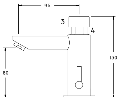
DIMENSIONES GENERALES
