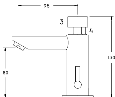
DIMENSIONES GENERALES
