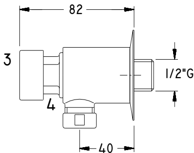
DIMENSIONES GENERALES
