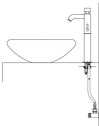
ESQUEMA TÍPICO DE INSTALACION
