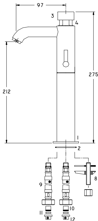
DIMENSIONES GENERALES
