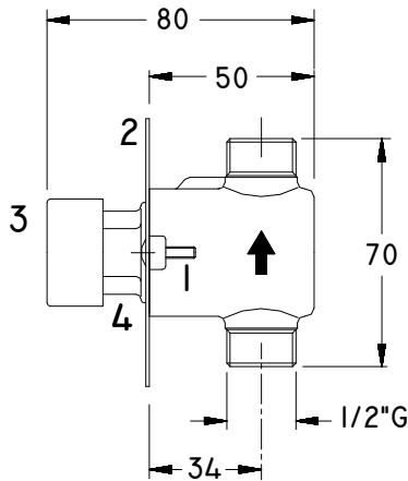
DIMENSIONES GENERALES
