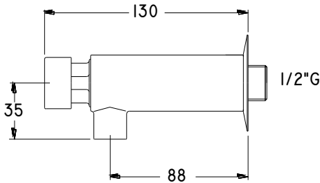
DIMENSIONES GENERALES
