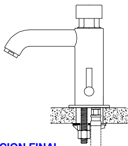
INSTALACION FINAL
