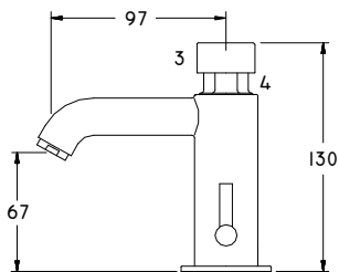
DIMENSIONES GENERALES
