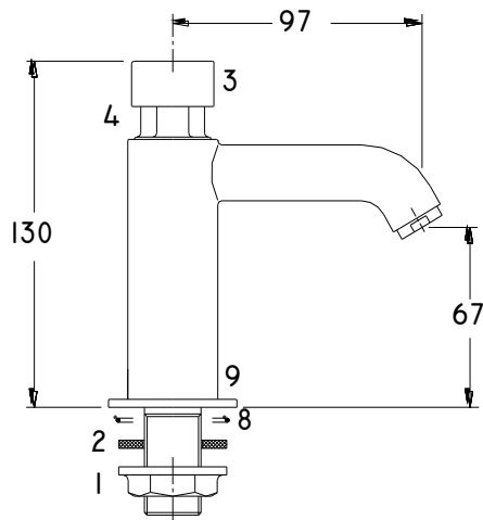
DIMENSIONES GENERALES
