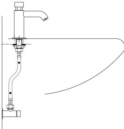
ESQUEMA TÍPICO DE INSTALACION
