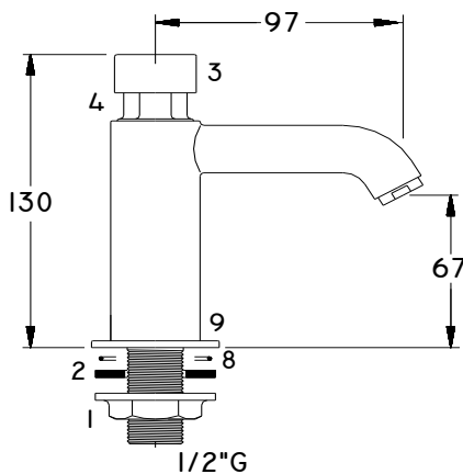
DIMENSIONES GENERALES
