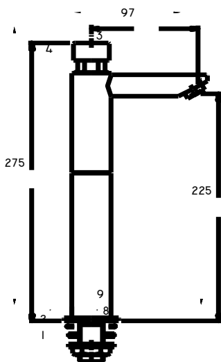
DIMENSIONES GENERALES
