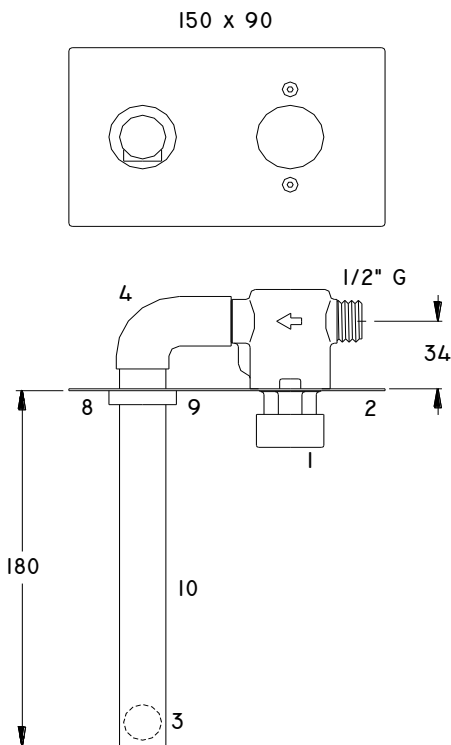
DIMENSIONES GENERALES
