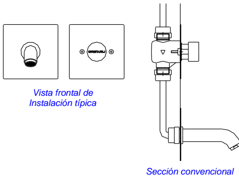
Sección convencional
