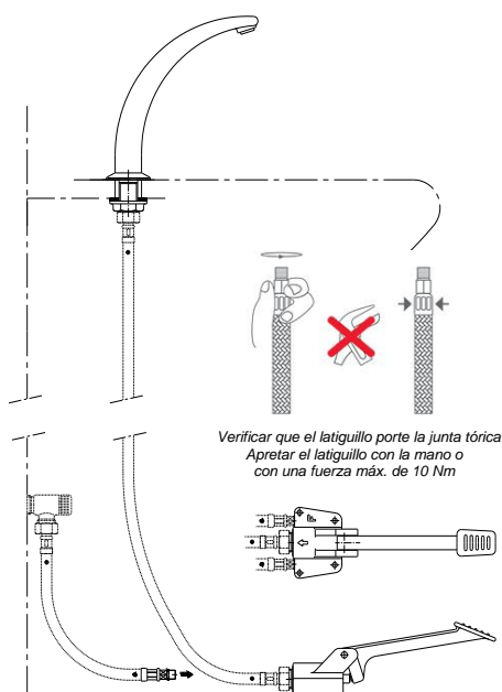
ESQUEMA TIPICO DE INSTALACION
