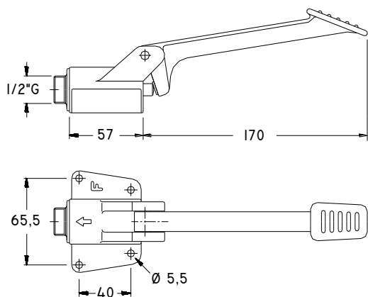
DIMENSIONES GENERALES
