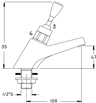
DIMENSIONES GENERALES
