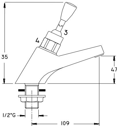
DIMENSIONES GENERALES
