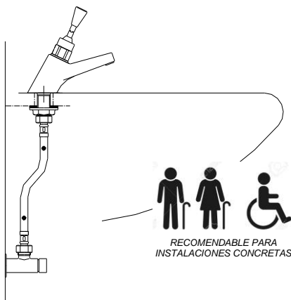
ESQUEMA TIPICO DE INSTALACION
