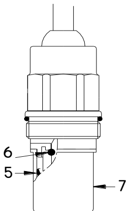
ROSCA M.29x1.5
