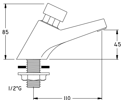
DIMENSIONES GENERALES
