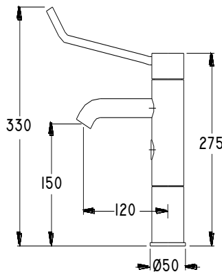
DIMENSIONES GENERALES
