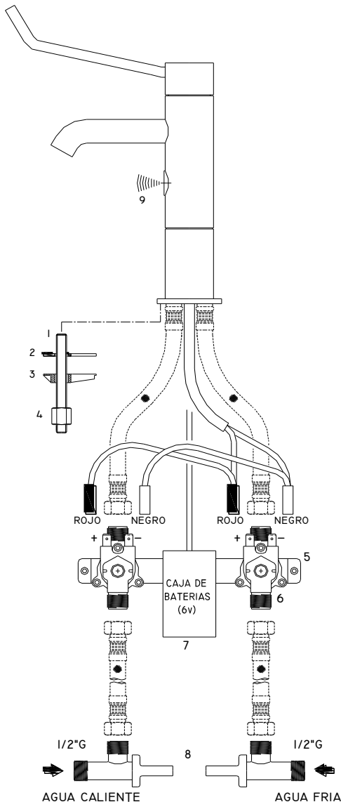
ESQUEMA DE CONEXIONES (ELECTRICA & HIDRAULICA)
