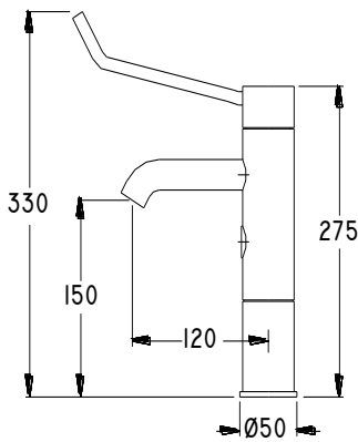
DIMENSIONES GENERALES
