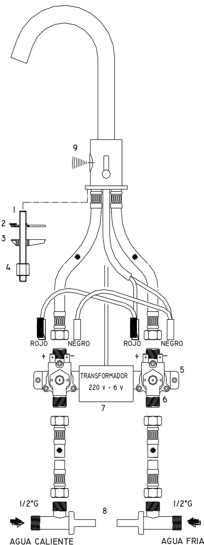
ESQUEMA DE CONEXIONES (ELECTRICA & HIDRAULICA)
