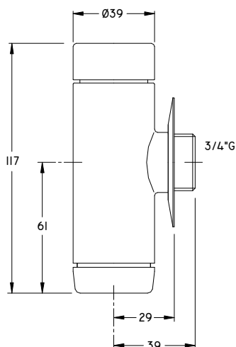
DIMENSIONES GENERALES
