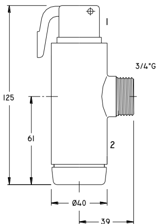
DIMENSIONES GENERALES
