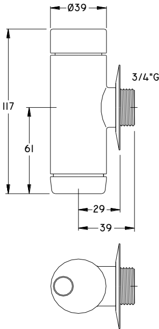
DIMENSIONES GENERALES
