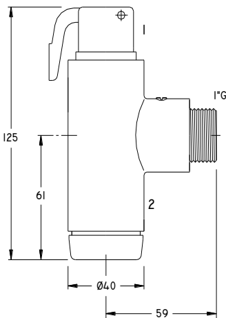
DIMENSIONES GENERALES
