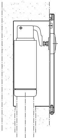
ESQUEMA TÍPICO DE INSTALACION
