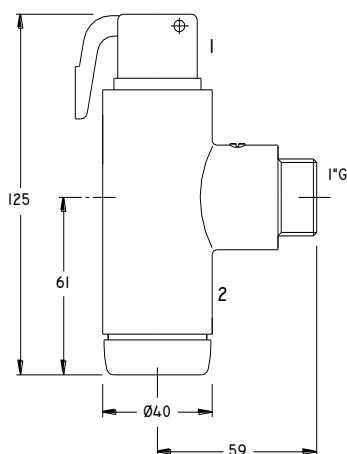
DIMENSIONES GENERALES
