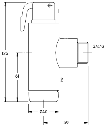
DIMENSIONES GENERALES
