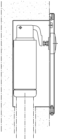
ESQUEMA TÍPICO DE INSTALACION
