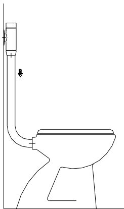
ESQUEMA TÍPICO DE INSTALACION
