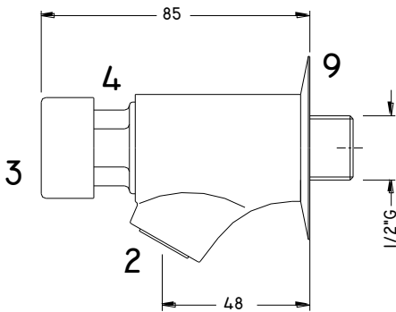
DIMENSIONES GENERALES
