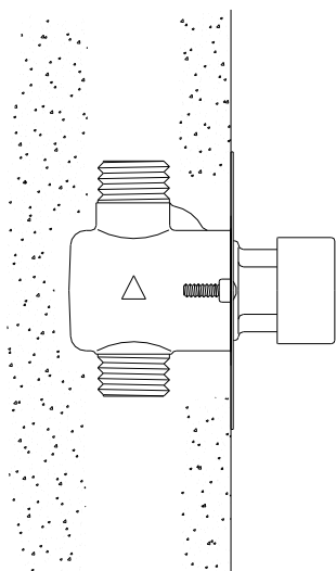
INSTALACION FINAL
