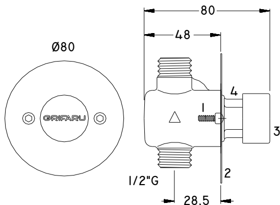
DIMENSIONES GENERALES
