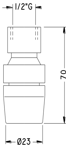
DIMENSIONES GENERALES Y COMPONENTES
