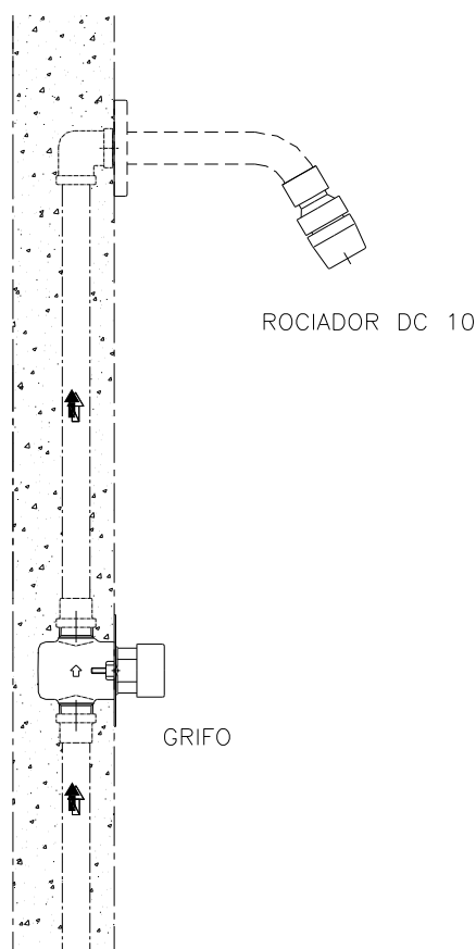
ESQUEMA DE INSTALACION TIPICA
