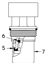
ROSCA M.29x1.5
