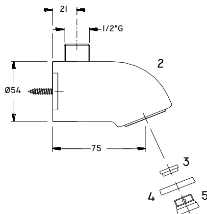
DIMENSIONES GENERALES Y COMPONENTES
